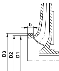
Fig.6: Section pompe RD
