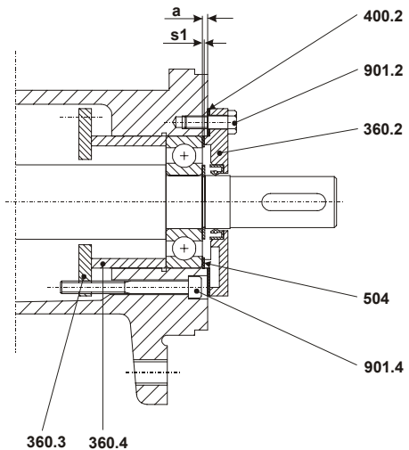
Fig.8 Sección para reglar bomba RG
