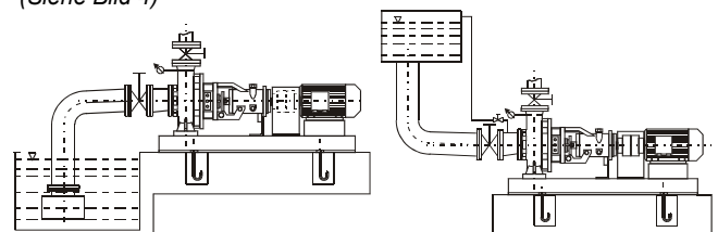
Bild 4: Rohrleitungsanschluss
