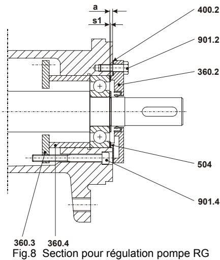
Fig.8 Section pour régulation pompe RG
