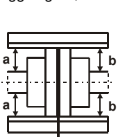
Fig. 2 Allineamento giunto
