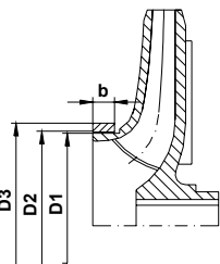
Fig. 6: Sezione pompe RD
