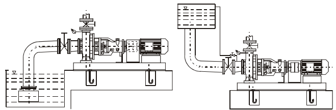
Fig.4 Fissaggio tubazioni
