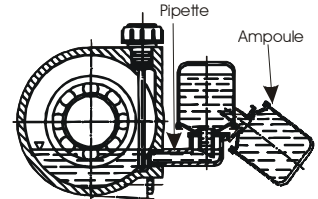
Fig.3: Graisseur
