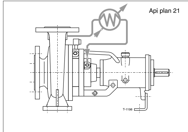
FLUSSAGGIO DALLA MANDATA CON SCAMBIATORE DI CALORE Recirculation from pump case though cooler to seal
