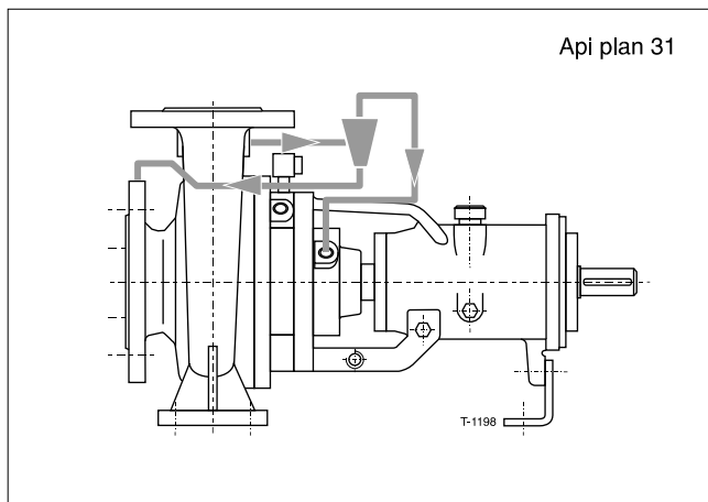
FLUSSAGGIO DALLA MANDATA CON CICLONE SEPARATORE Recirculation from pump case through cyclone separator to seal
