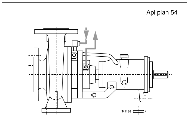
FLUSSAGGIO DELLA TENUTA MECCANICA DOPPIA DA FONTE ESTERNA CON LIQUIDO PULITO Circulation of clean liquid to double seal from an external circulation system
