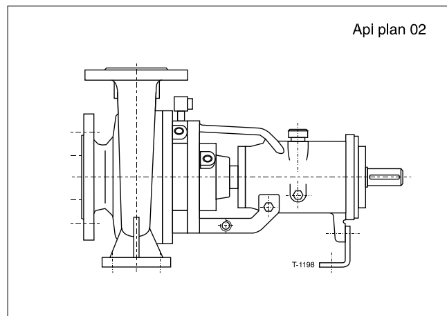
FLUSSAGGIO DALL'INTERNO Internal recirculation from pump discharge to seal
