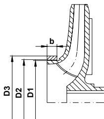
Fig.6: Sezionne pompe RB
