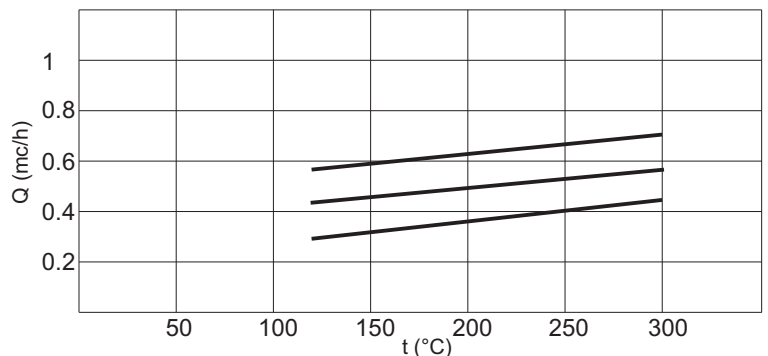
Flussaggio camera di raffreddamento esecuzione H Cooling chamber flushing H exec.
