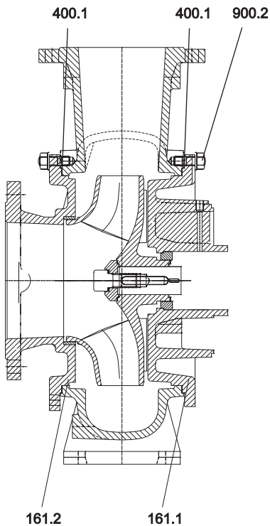
POMPA TIPO: 150-35, 200-35, 250-35
