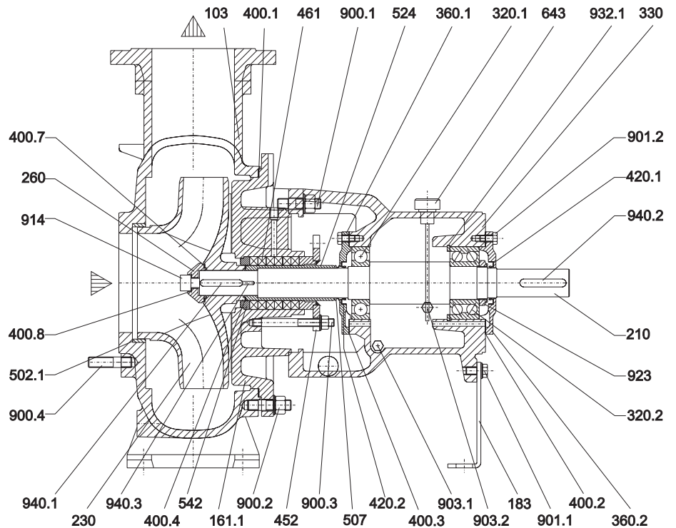
POMPA TIPO: 100-25, 125-25, 80-31, 125-31
