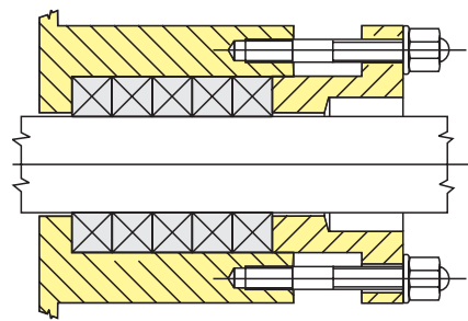
Tenuta a baderna senza flussaggio. Gland packing without flushing. "B" execution.
